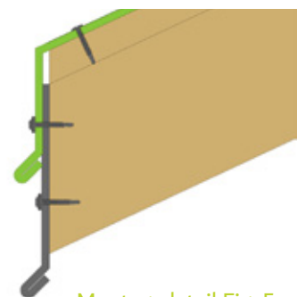
Montagedetail Fig. 5
