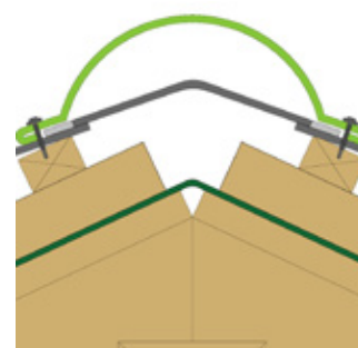
Montagedetail Fig. 67
