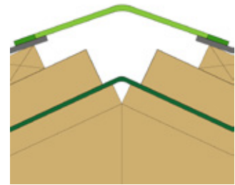
Montagedetail Fig. 65
