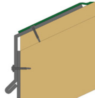
Montagedetail Fig. 10
