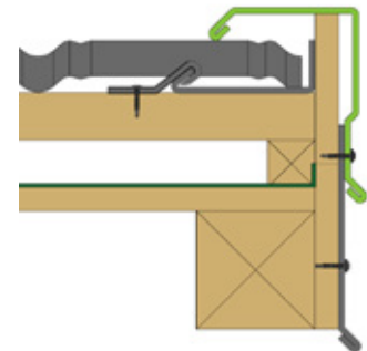
Montagedetail Fig. 57
