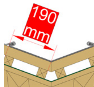
Montagedetail Fig. 22
