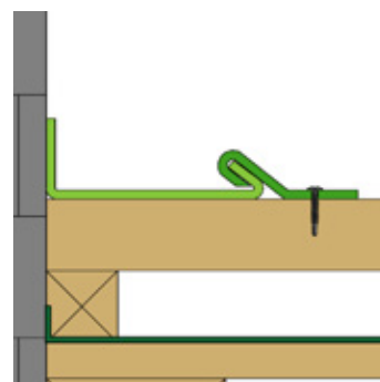
Montagedetail Fig. 31
