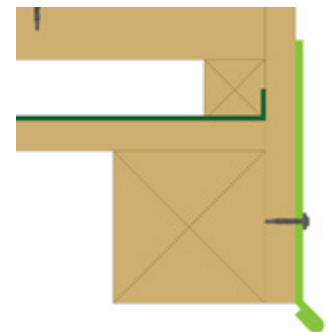
Montagedetail Fig. 51
