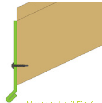
Montagedetail Fig. 4
