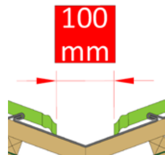
Montagedetail fig. 37
