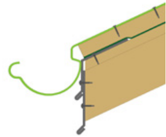
Montagedetail Fig. 15
