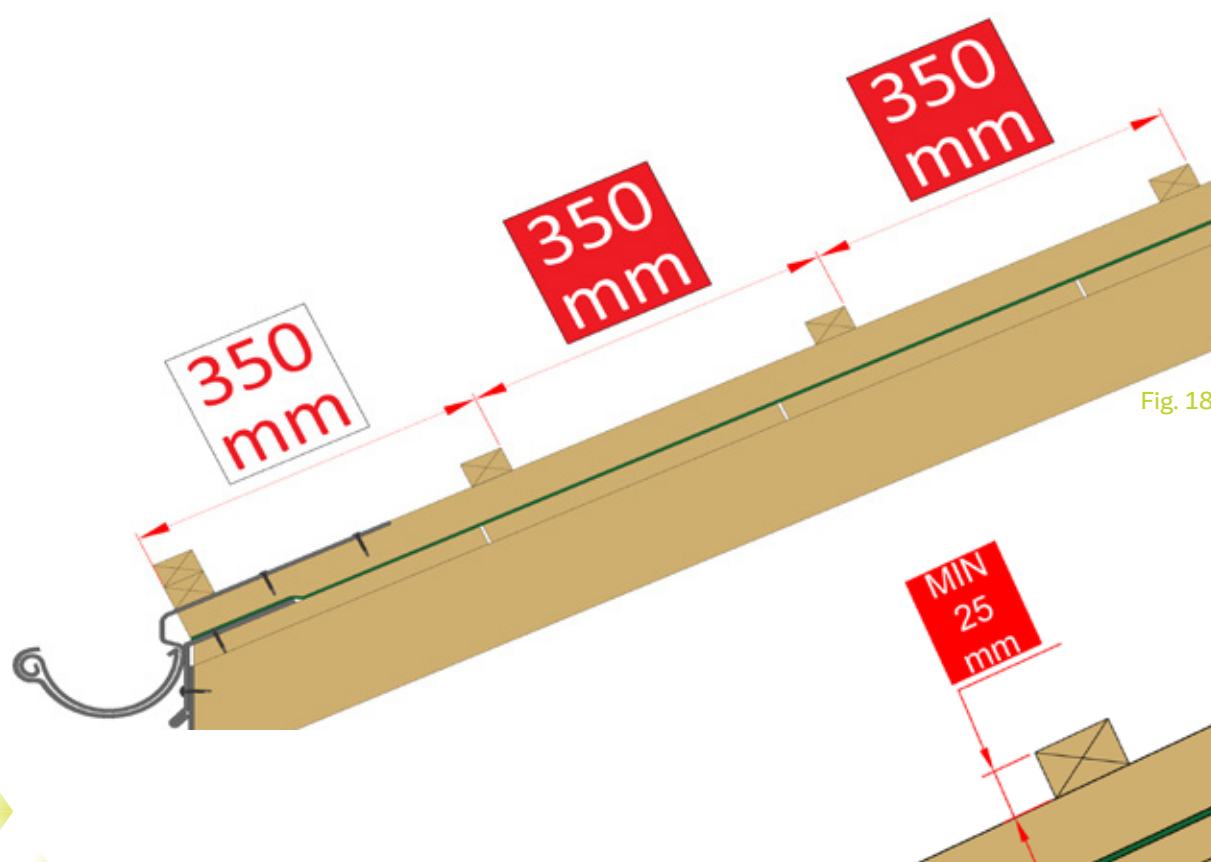
Montagedetail Fig. 18
