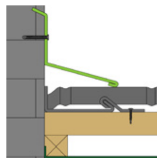
Montagedetail Fig. 49
